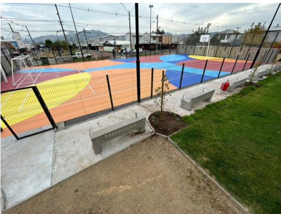
IMAGEN 18 MULTICANCHA POBLACIÓN DON SEBASTIÁN.
