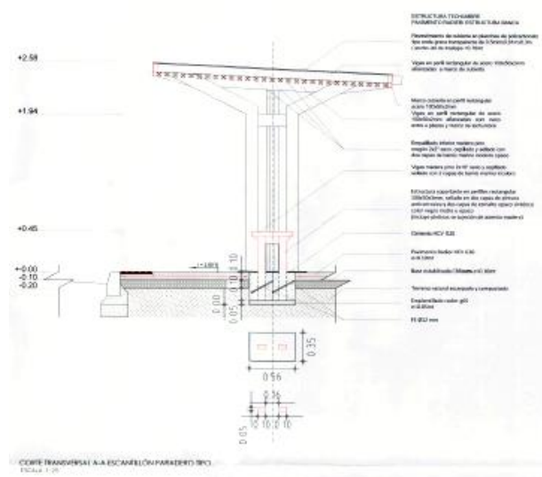
IMAGEN 35 PLANIMETRÍA PARADEROS URBANOS.
