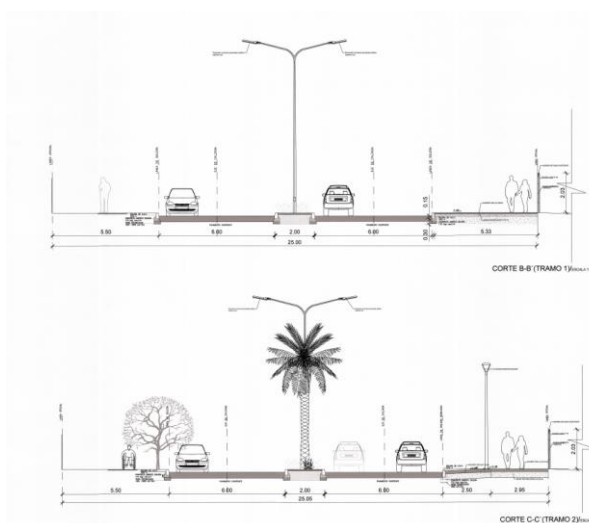
IMAGEN 31 PLANIMETRÍA DEL PROYECTO MEJORAMIENTO VEREDA SUR AVENIDA DOCTOR FAÚNDEZ.
