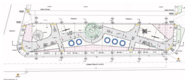
IMAGEN 36 PLANIMETRÍA MEJORAMIENTO ÁREA VERDE LOS OLIVOS DE VILUCO.
